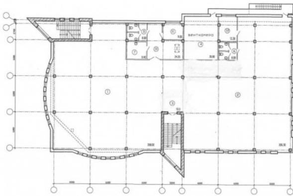
ПЛАН 2 ЭТАЖА
